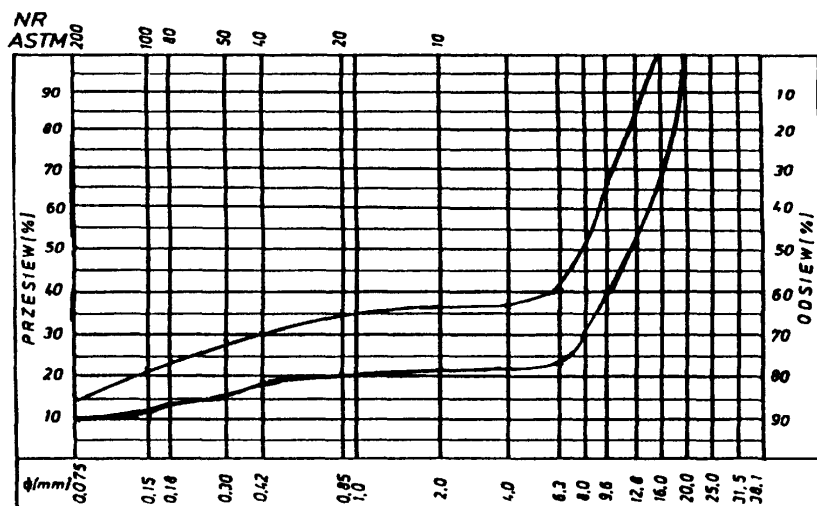
Rys. 5. Krzywe graniczne uziarnienia mieszanki mineralnej 020 mm o nieciągłym uziarnieniu do warstwy ścieralnej z betonu asfaltowego dla KR 3
