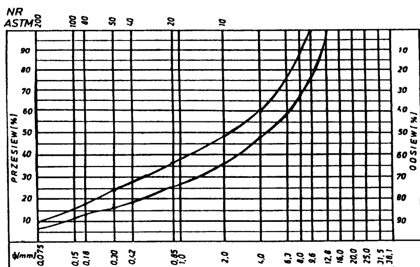
Rys. 7. Krzywe graniczne uziarnienia mieszanki mineralnej 012,8 mm do warstwy ścieralnej z betonu asfaltowego dla KR 3
